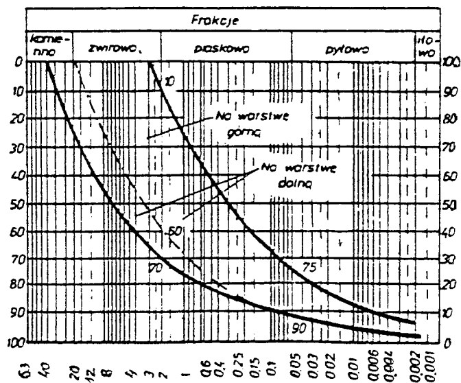
Rysunek 2. Obszar uziarnienia optymalnych mieszanek gliniasto-żwirowych
