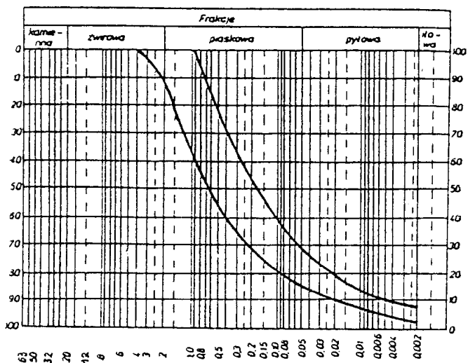
Rysunek 1. Obszar uziarnienia optymalnej mieszanki gliniasto-piaskowej
