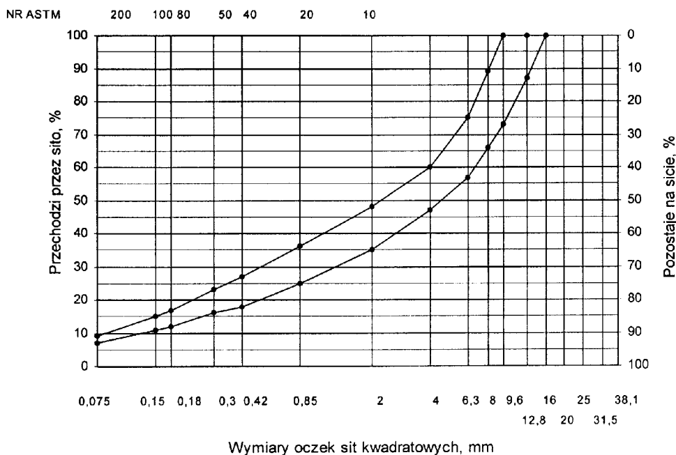
graniczne uziarnienia mieszanki mineralnej BA od 0 do 16 mm do warstwy ścieralnej nawierzchni drogi o obciążeniu ruchem od KR3 do KR6
