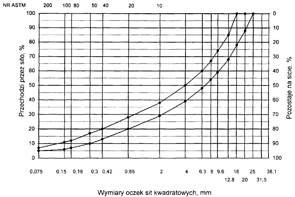
graniczne uziarnienia mieszanki mineralnej BA od 0 do 20 mm do warstwy ścieralnej nawierzchni drogi o obciążeniu ruchem od KR3 do KR6
