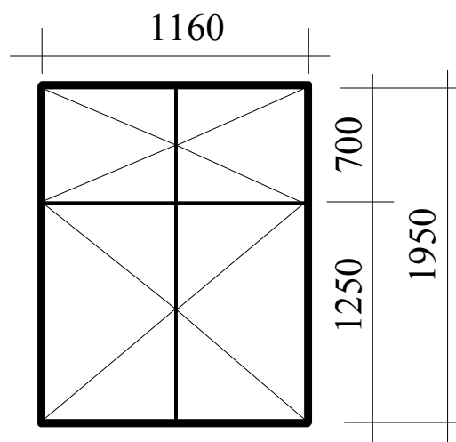
TYP B
