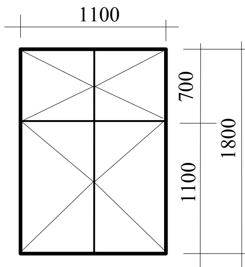
TYP D
