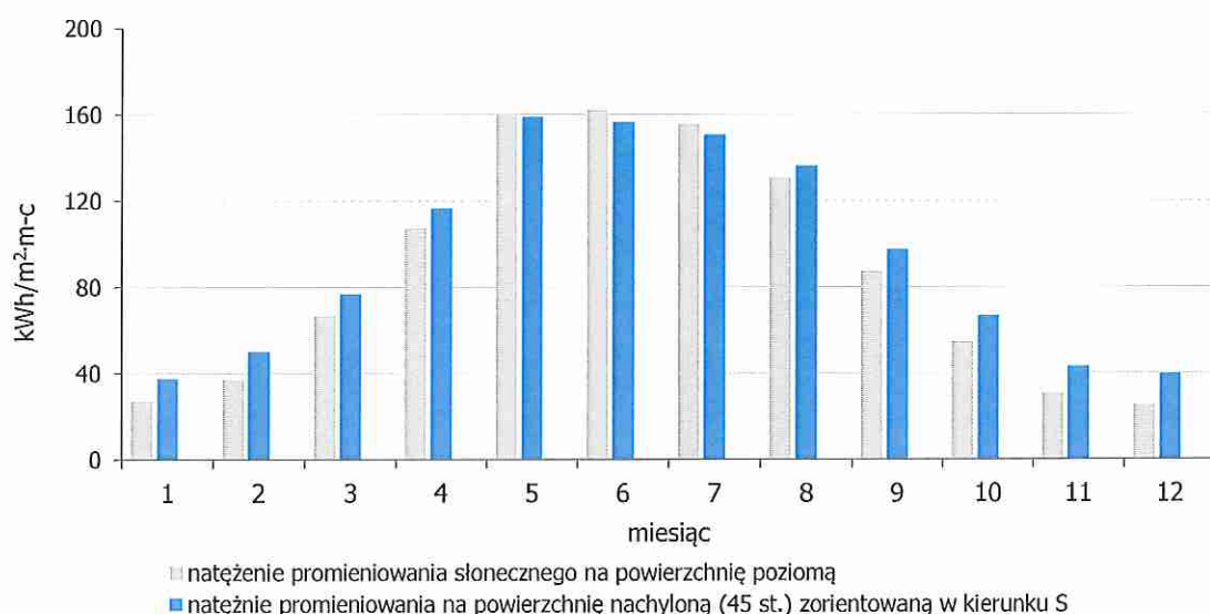
Rysunek 4-7 Energia promieniowania słonecznego na rozpatrywanym obszarze (natężenie promieniowania na powierzchnię poziomą oraz nachyloną pod kątem 45° dla danego miesiąca w ciągu roku)
