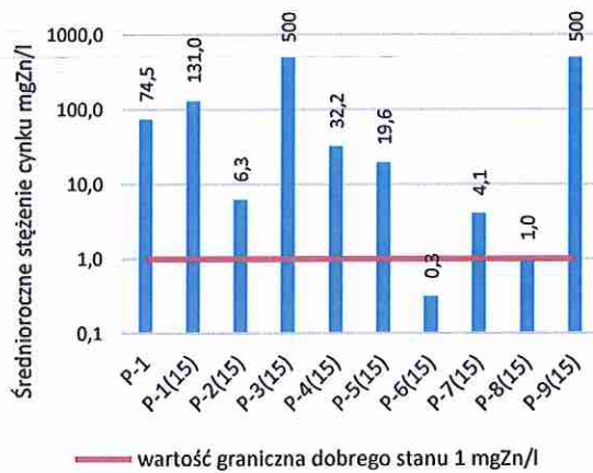
Wykres 10. Średnioroczne stężenia cynku w piezometrach monitorujących wody podziemne w rejonie miejsca magazynowania szlamów cynkowych przy II Kompleksie HMN „Szopienice” SA w likwidacji w roku 2015
