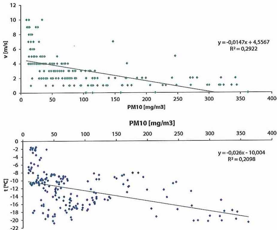
Wykres 21. Współczynnik korelacji Pearsona między stężeniem PM10 na stacji PMS w Sosnowcu a temperaturą powietrza i prędkością wiatru dla epizodu z okresu 21-28 stycznia 2010 r.
