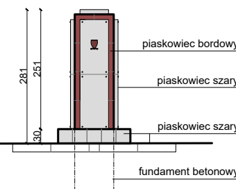
WIDOK PÓLNOCCY tylny w stronę Urzędu Miasta
